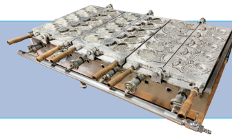
たい焼き機 (15個) サイズ/W920×D660 H180 ※ ガス使用量:1.7kg/h
