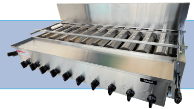
荒磯(ガス赤外線グリラー) サイズ/W1130×D600 H260 ※ ガス使用量/1.24kg/h
