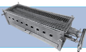
焼き鳥コンロ サイズ/W710×250 H200 ※ ガス使用量/0.63kg/h
