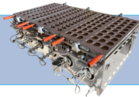
たい焼き機 (ミニ) サイズ/W1000×D700 ※ H310 ※ ガス使用量:0.7kg/h
