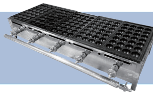
たこ焼き機(150個) サイズ/W1000×D480 H200 ※ ガス使用量/1.5kg/h
