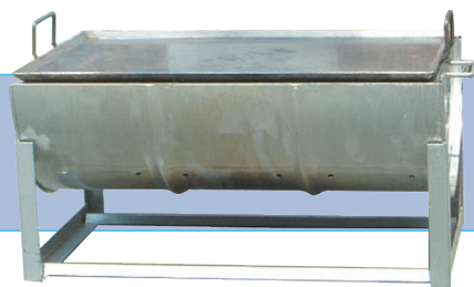
バーベキューセット(ドラム缶ハーフ)
